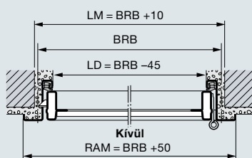
Külső szerelésű, kifelé nyíló
