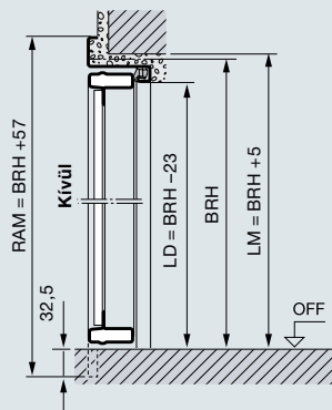
Belső szerelésű, befelé nyíló
