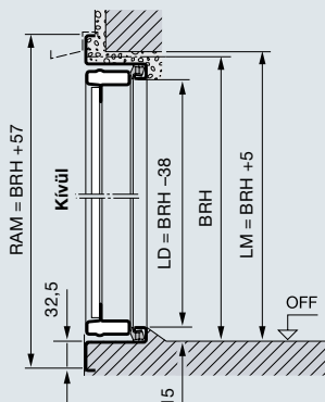
1-szárnyú, küszöbkel
