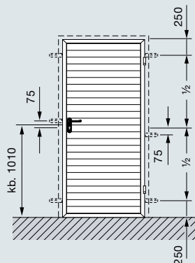
1-szárnyú, küszöb nélkül
