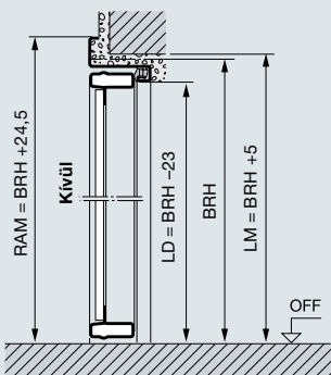
Külső szerelésű, kifelé nyíló
